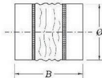
Giunti antivibranti risvoltati Esecuzione in lamiera zincata Anti-vibration joints made of folded-up galvanized sheet metal
